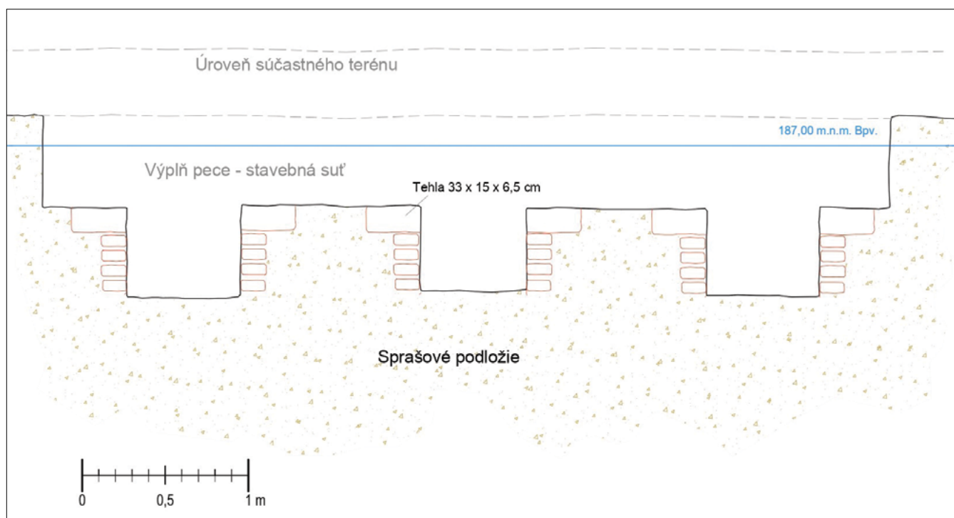
Obr. 5: Priečny rez A vnútri tehliarskej pece. Podľa P. Nagya kreslila D. Nagyová
