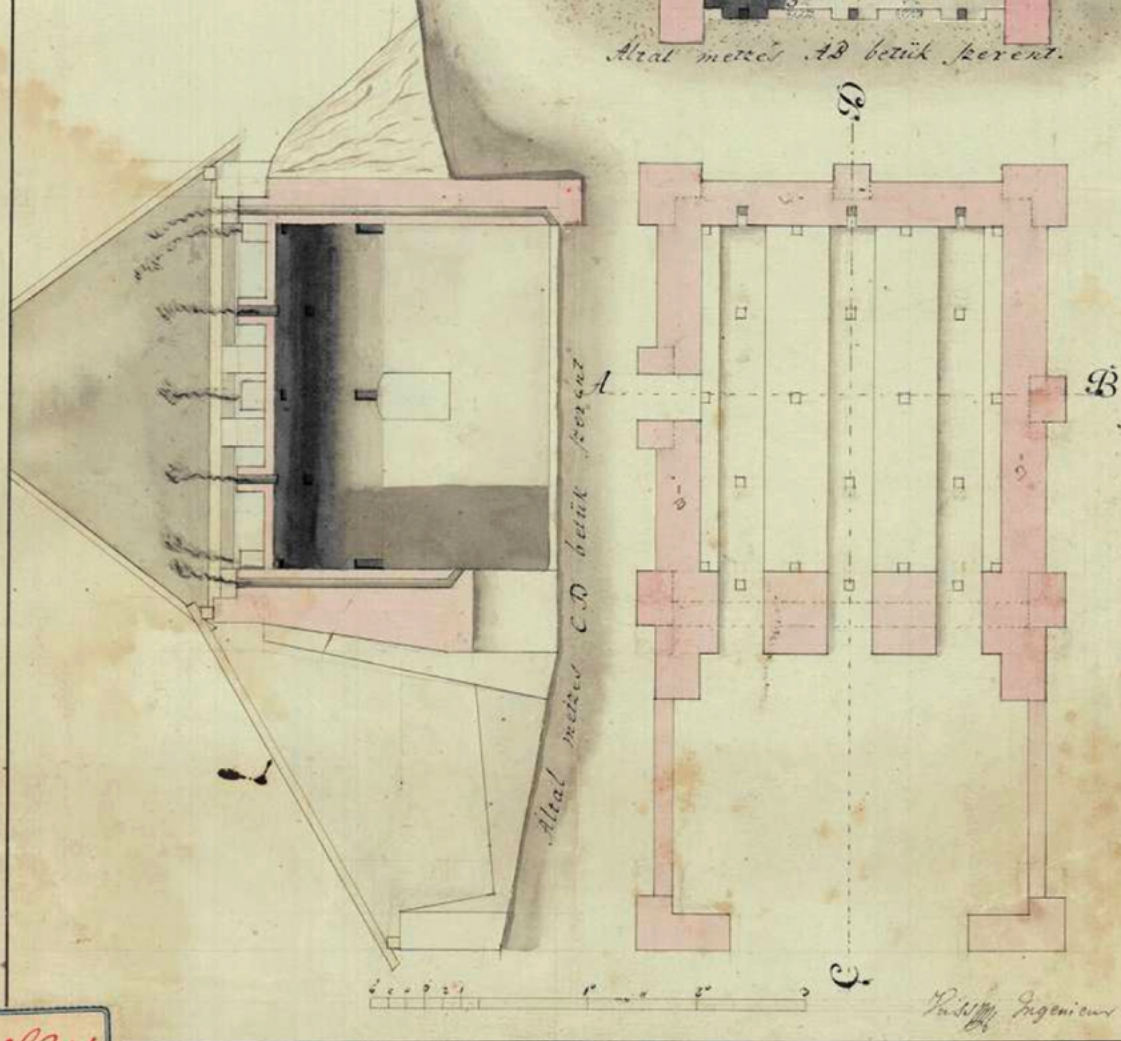
Obr. 9: Plán tehliarskej pece z Keszthely. Podľa https://maps.hungaricana.hu/en/MOLTervtar/6798/view/?pg=0&bbox=-1889%2C-4544%2C5350%2C-345
