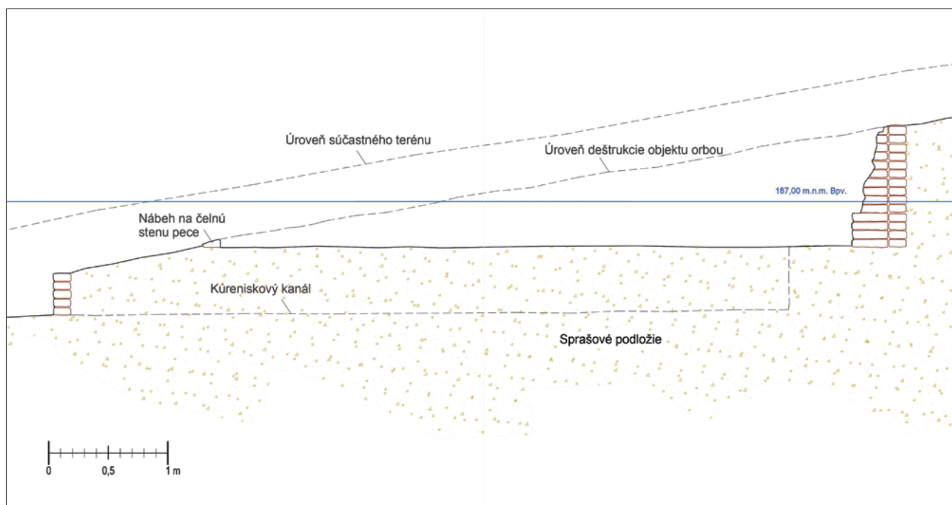
Obr. 6: Pozdĺžny rez B vnútri tehliarskej pece. Podľa P. Nagya kreslila D. Nagyová
