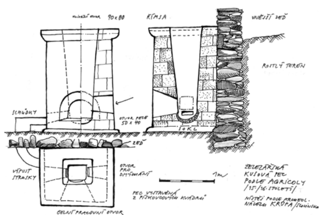
Obr. 25: Nerealizovaný návrh železářské pece, jež měla být postavena v objektu Šlakhamru. Na rekonstrukci Brdíčkovy mlýna a jeho přeměně do současné podoby se poměrně zásadní měrou podílel
