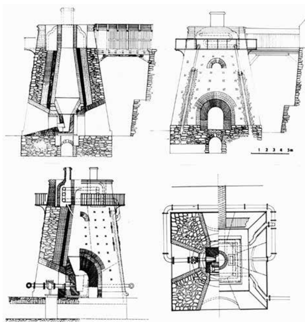
Obr. 29: Velká pec v Josefově, rekonstrukce – pohled a řezy zhotovené JM. Dobře kreslil, ať již se jednalo o mapky, plány, rekonstrukce staveb, zobrazení sbírkových předmětů do evidenčních karet, obrázky pro děti. Zhotovoval nám trička s malovanými obrázky, jaká nikdo jiný neměl, rozličné vlajky (možno shlédnout při táborech v Josefově). Vyřezával rytíře a setrval doplnoval figurami domácí betlém – má i hamernickou a hornickou část
