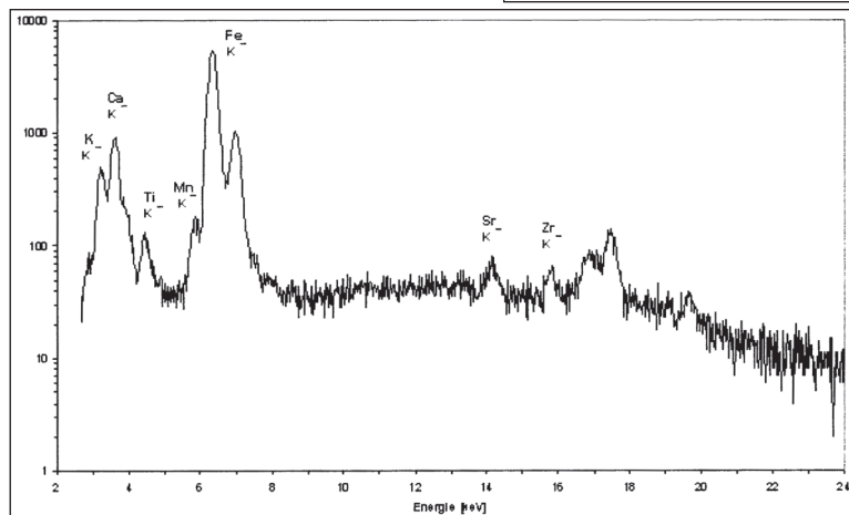
Obr. 12: XRF spektrum povrhu strusky 104/5
