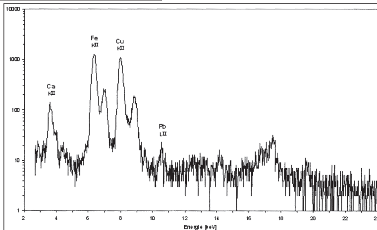
Obr. 13: XRF spektrum povrhu strusky 119/6
