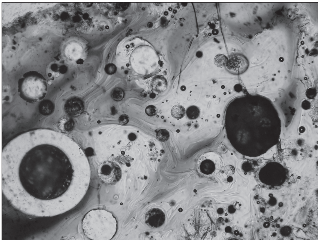
Obr. 8: Fluidální mikrostruktura s kruhovými póry, 10x, PPL
